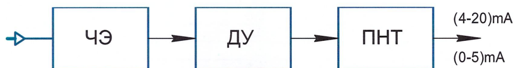
Рисунок 1 - Структурная схема датчика давления ДДМ
