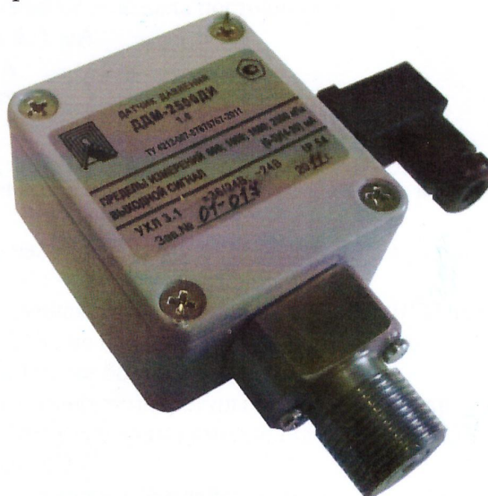
Фото 1 - Фотография общего вида датчика давления ДДМ
